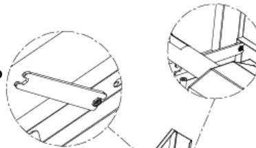
Podkładka płaska M6 Ilość: 3 szt.
