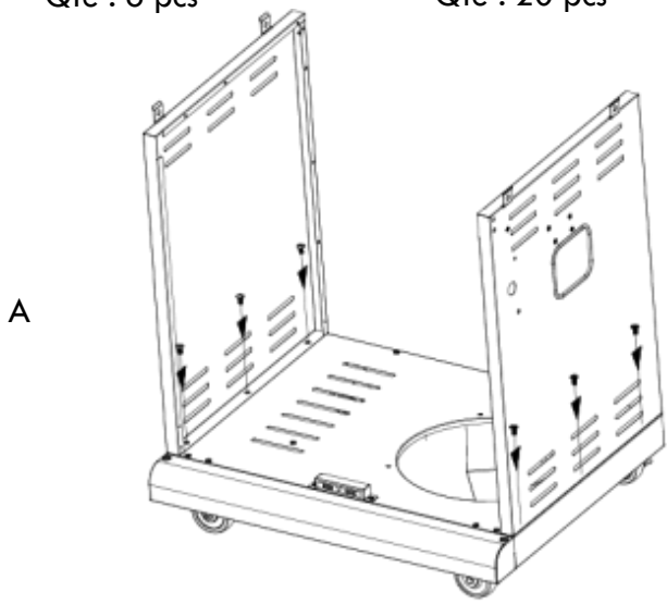
Vis M6 x 13 Qté : 6 pcs
