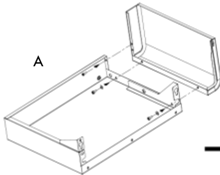
Podkładka płaska M6 Ilość: 3 szt.
