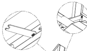
M4x10 Sechskantschraub Anz: 1 Stück
